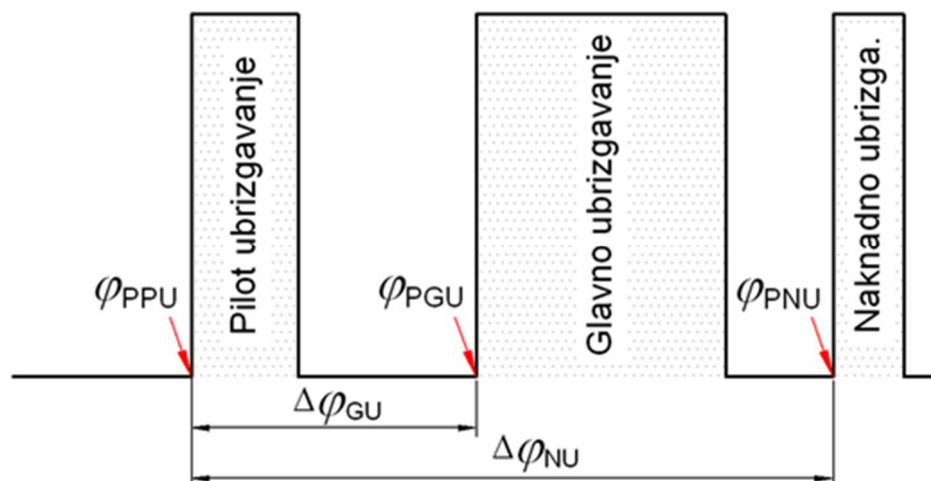
Slika 8.48. Podijeljeno (višestruko) ubrizgavanje goriva
