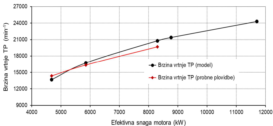
Slika 7.12 Usporedba brzine vrtnje TP za različita opterećenja motora
