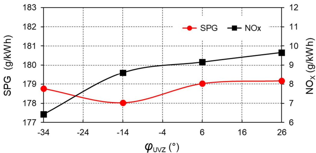
Slika 8.40. Utjecaj ranijeg ZUV na SPG i emisiju NO_x pri 100% P_n
