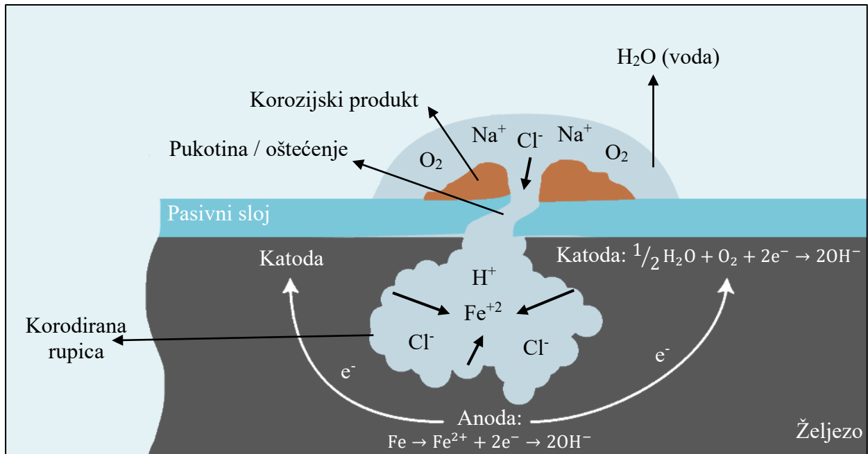
Slika 5.10. Rupičasta korozija
