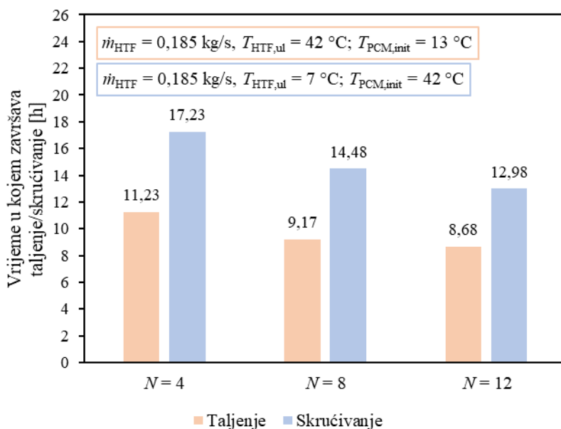
Slika 8.7. Usporedbe vremena u kojima završavaju taljenje/skrucivanje dobivenih numeričkim proračunima za analizirane brojeve lamela
