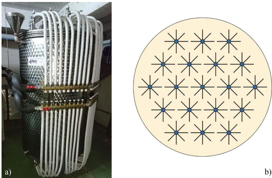
Slika 2.1. Latentni spremnik topline cijevne konfiguracije s lamelama, a) razmatrani latentni spremnik topline, b) konfiguracija cijevi i lamela unutar spremnika
