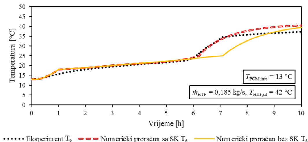
Slika 7.6. Vremenske promjene temperatura akumulatora topline prilikom taljenja dobivene eksperimentalno i numerički s i bez utjecaja slobodne konvekcije na poziciji T_6
