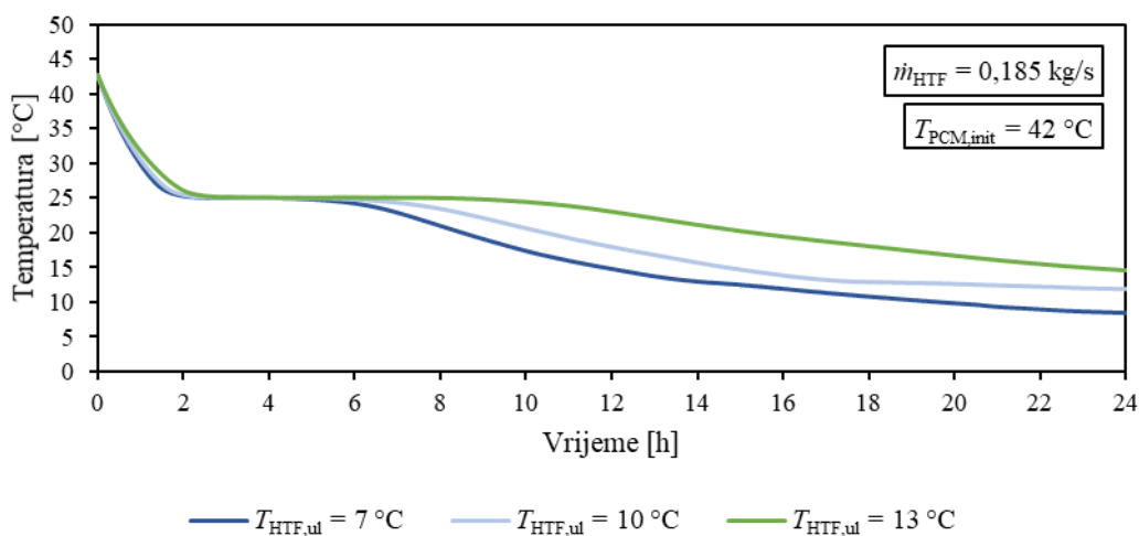
Slika 4.6. Vremenske promjene temperatura akumulatora topline prilikom korištenja topline dobivene eksperimentalnim mjerenjima na mornoj poziciji T 2 za različite ulazne temperature fluida prijenosnika topline
