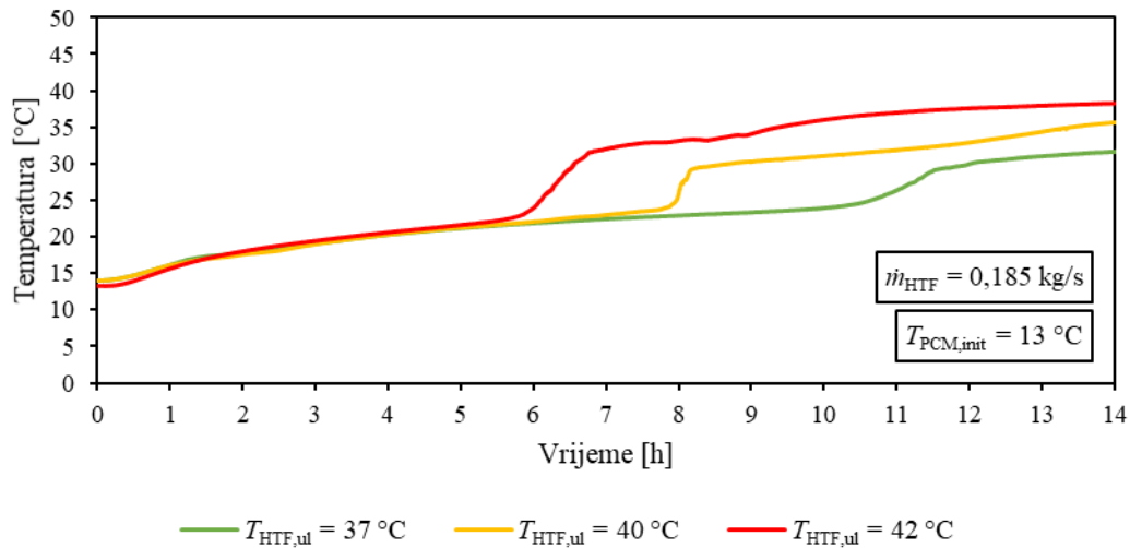
Slika 4.2. Vremenske promjene temperatura akumulatora topline prilikom spremanja topline dobivene eksperimentalnim mjerenjima na mjernoj poziciji T_6 za različite ulazne temperature fluida prijenosnika topline
