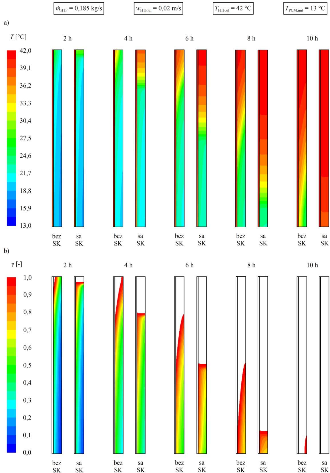
Slika 7.7. Usporedba raspodjela temperatura (a) i udjela kapljevite faze (b) u središnjoj ravlini između lamela prilikom taljenja akumulatora topline, dobivenih numeričkim proračunima s i bez slobodne konvekcije u proračunskim vremenima 2, 4, 6, 8 i 10 h
