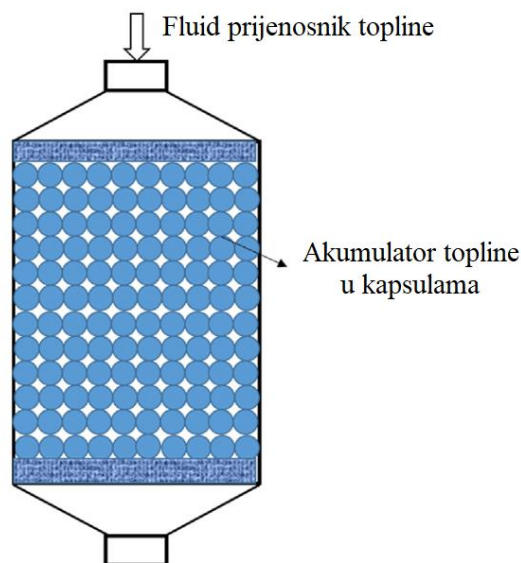
Slika 1.2. Latentni spremnik topline s akumulatorom topline u kapsulama [28]
