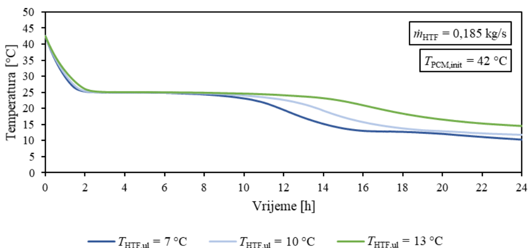
Slika 4.7. Vremenske promjene temperatura akumulatora topline prilikom korištenja topline dobivene eksperimentalnim mjerenjima na mornoj poziciji T 5 za različite ulazne temperature fluida prijenosnika topline
