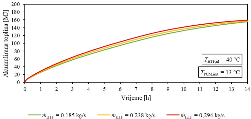
Slika 4.14. Vremenske promjene akumuliranih toplota prilikom spremanja topline dobivene rezultatima eksperimentalnih mjerenja za različite masene protoke fluida prijenosnika topline
