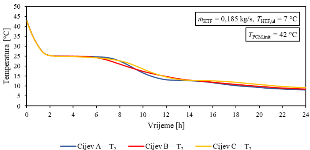
Slika 3.12. Vremenske promjene temperatura akumulatora topline prilikom skrućivanja na poziciji T_2 dobivene eksperimentalnim mjerenjima na različitim cijevima
