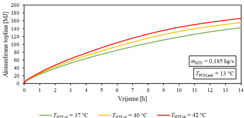
Slika 4.4. Vremenske promjene akumuliranih topline prilikom spremanja topline dobivene rezultatima eksperimentalnih mjerenja za različite ulazne temperature fluida prijenosnika topline
