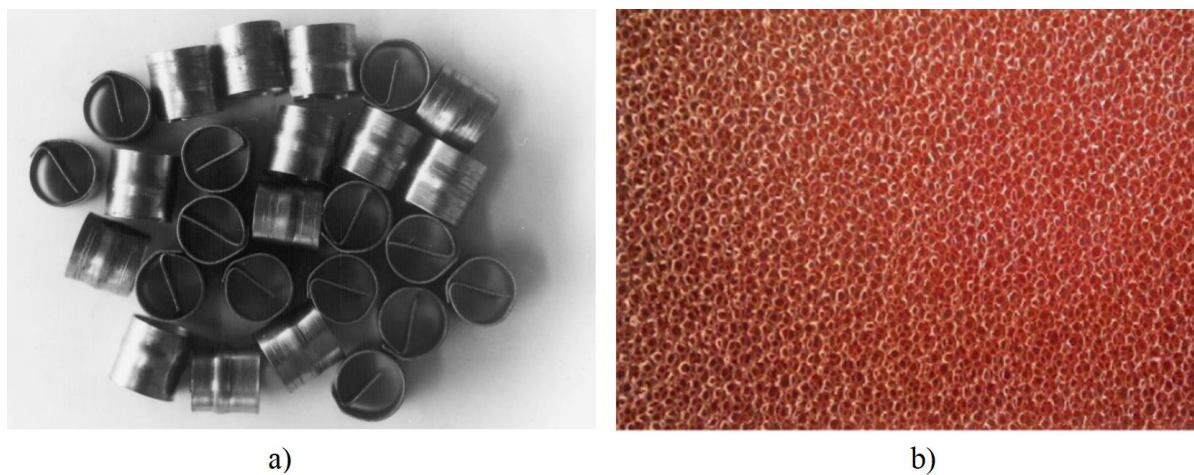
Slika 1.6. Primjer dodavanja dobro provodljivih elemenata u akumulator topline u svrhu poboljšanja njegove toplinske vodljivosti, a) metalni prstenovi [50], b) bakrena pjena [28]
