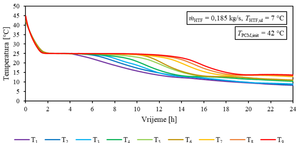
Slika 3.14. Vremenske promjene temperatura akumulatora topline prilikom skrućivanja oko središnje cijevi B dobivene eksperimentalnim mjerenjima u definiranom mjernom polju
