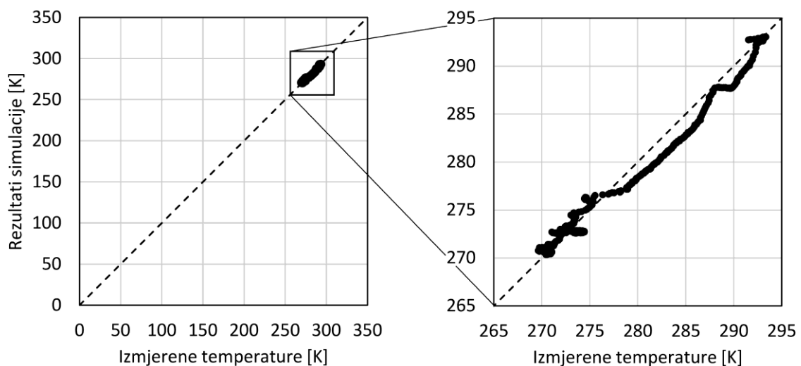
Slika 5.7 Usporedba izlazne temperature isparivača izračunate numeričkom simulacijom detaljnim modelom isparivača i eksperimentalnih mjerenja u prijelaznim uvjetima rada
