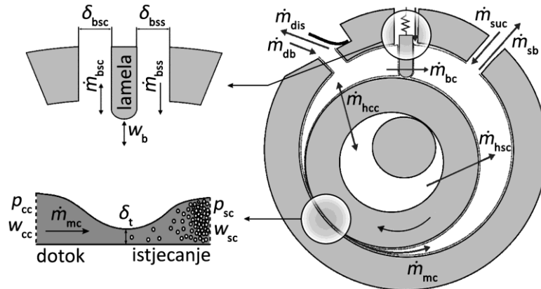
Slika 3.7 Maseni protoci na kompresoru s rotirajućim klipom, prerađeno iz Rocha (2019)
