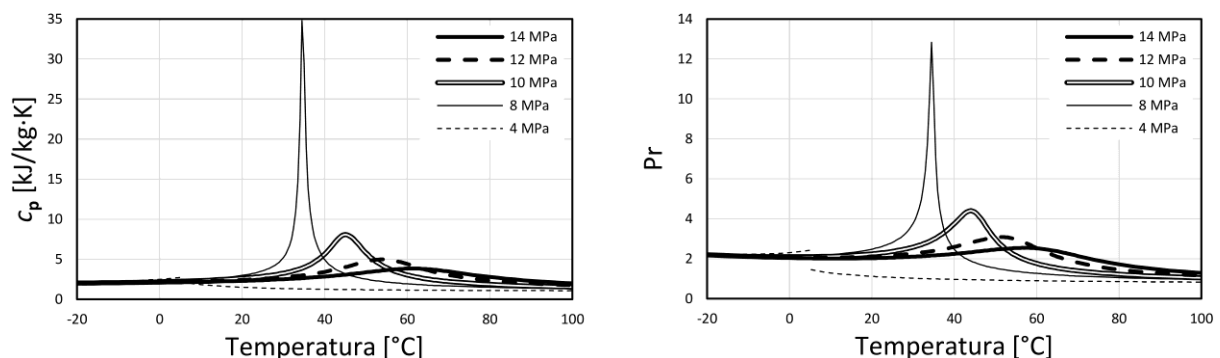
Slika 2.3 Izobarna specifična toplota CO 2 (lijevo) i Prandtllov broj (desno)
