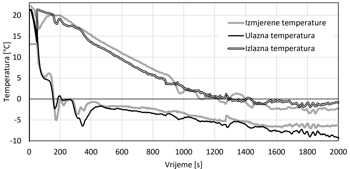
Slika 5.19 Usporedba izračunatih i izmjerenih temperatura radne tvari na ulazu i izlazu isparivača
