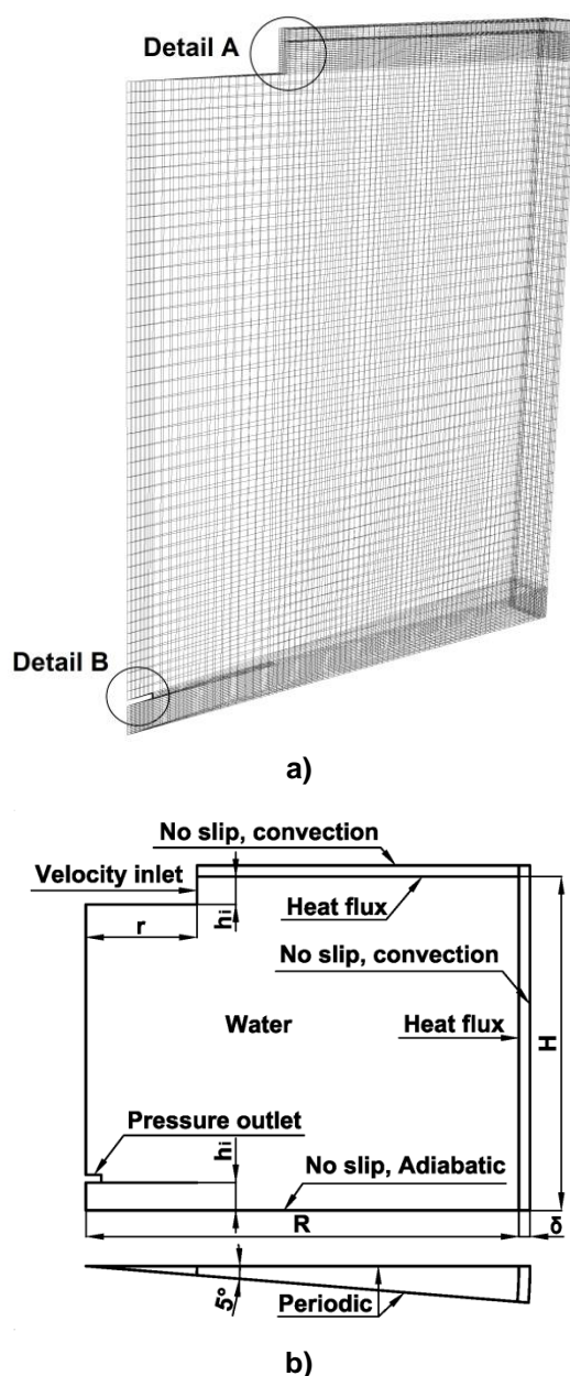
Slika 4.31. Domena s radialnim difuzorom za proces punjenja: a) umrežena domena, b) domena s rubnim uvjetima, [97]
