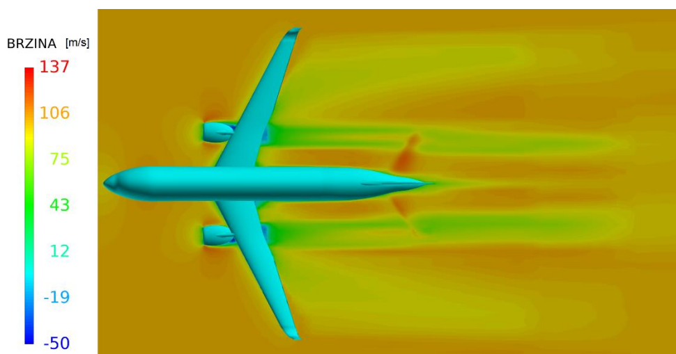
Slika 3.52 Brzine - Pogled od gore- Presjek 2 - 100 m/s i 70^\circ
