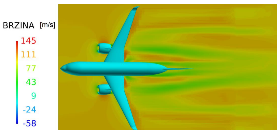
Slika 3.53 Brzine - Pogled od gore- Presjek 2 - 100 m/s i 15^\circ
