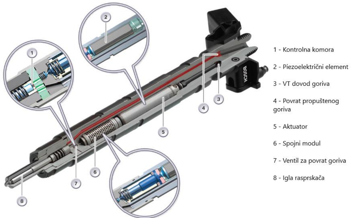
Slika 3.12 Presjek piezoelektriinog rasprskaa goriva s naznaenim glavnim dijelovima [14]
