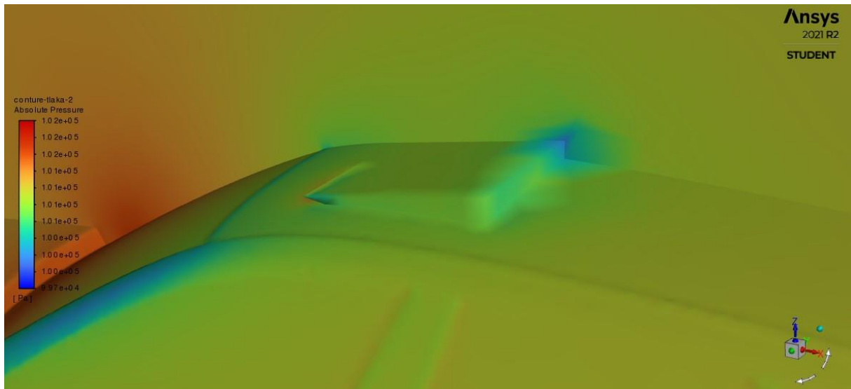
Slika 8.4. Detalj konture apsolutnog tlaka kod krovnog prozora
