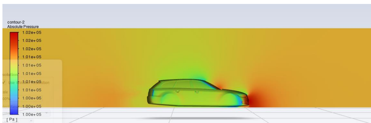
Slika 5.1. Konture apsolutnog tlaka zraka na presječnoj ravnini
