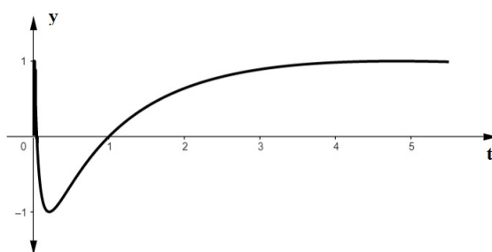
Slika 5.4. Grafički prikaz funkcije f(t)=\sin(\ln t) ; Izvor; Izrada autora
