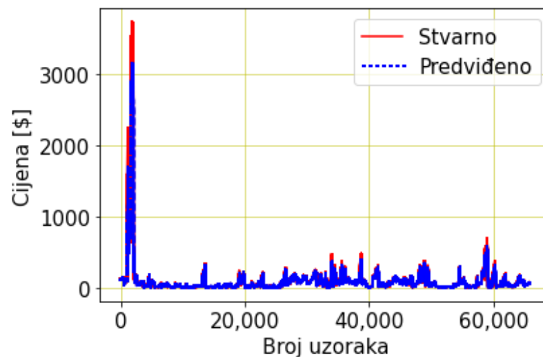
Slika 5.3 Prikaz svih predviđanja modela
