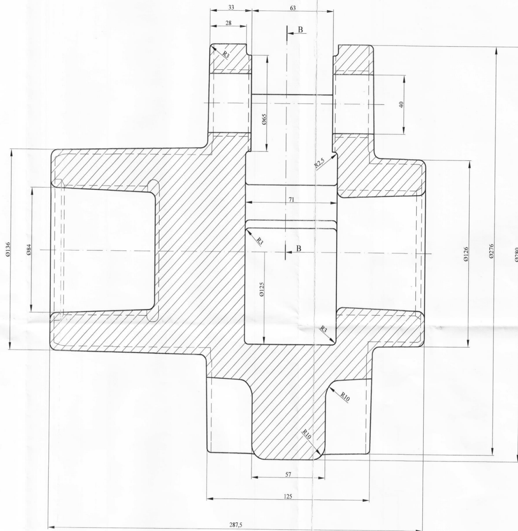
Presjek A-A
