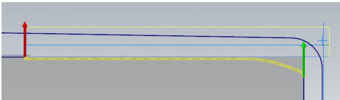
Slika 6.46 Smjer kretanja alata za šesti zahvat
