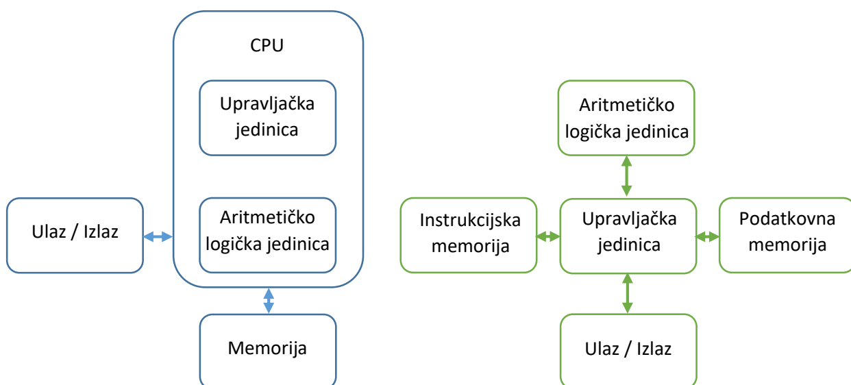
Slika 2.4. Von Neumannova (lijevo) i Harvarska arhitektura (desno).
