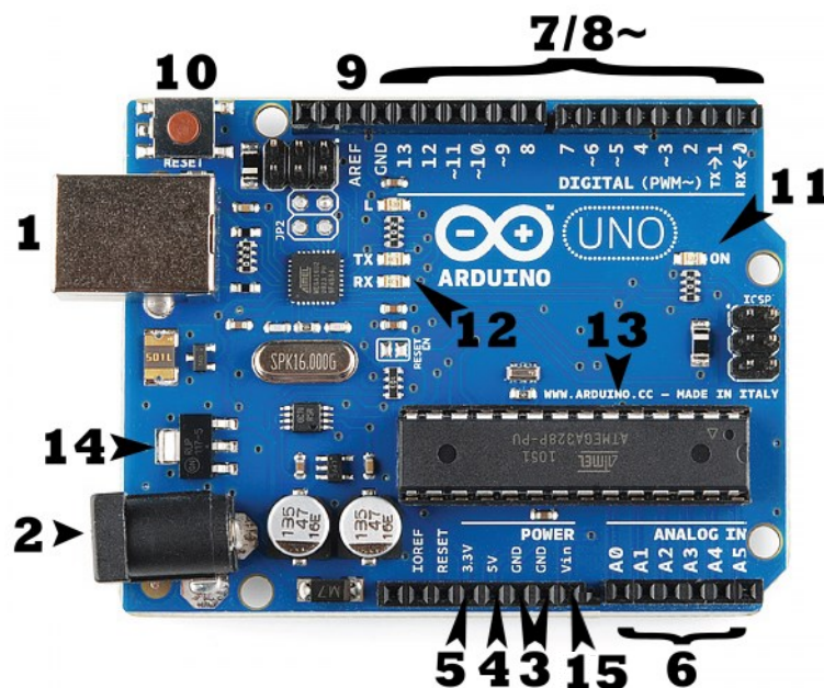
Slika 2.1. Arduino Uno razvojna pločica s označenim dijelovima [2].
