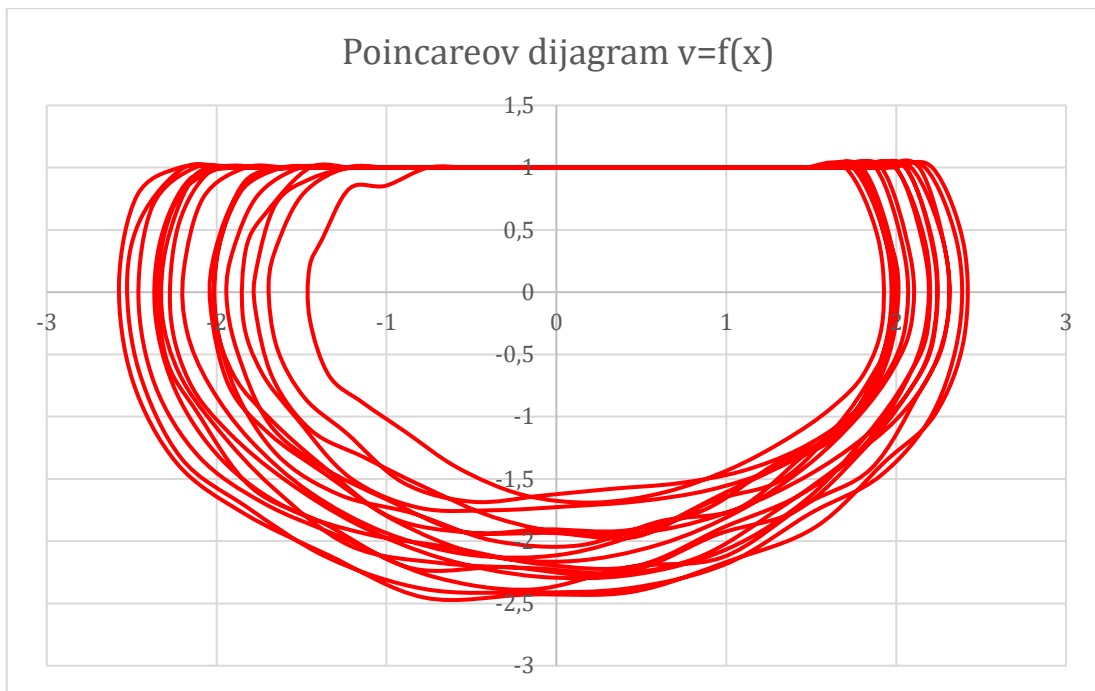
Slika 6.15. Poincareov dijagram za \Omega=1,22
