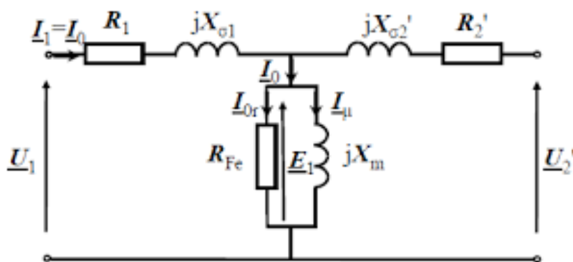
Slika 5.1. Nadomjesna shema transformatora
