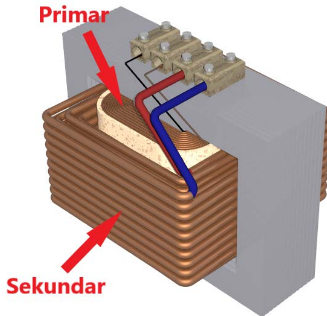
Slika 3.3. Model transformatora
