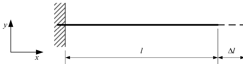
Slika 5.1 – Geometrija jednodimenzijuskog štapa opterećenog aksijalnim pomakom.
