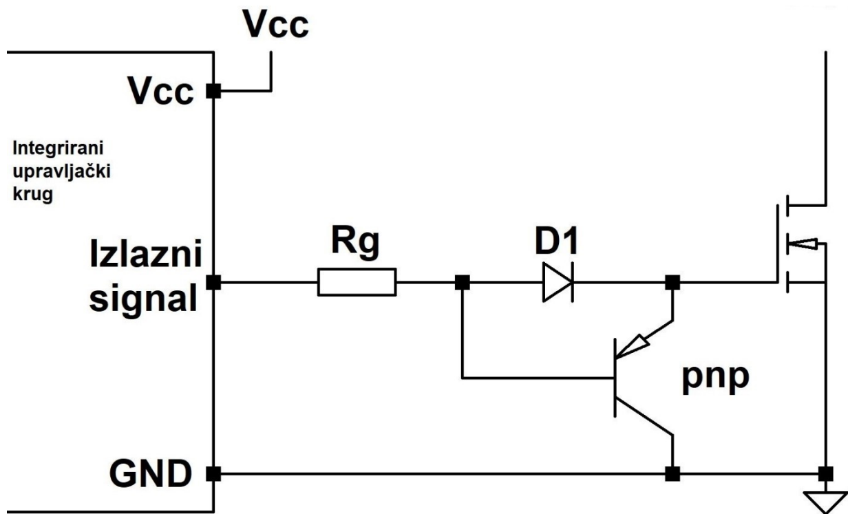
Slika 5.10. Upravljački sklop s pnp bipolarnim tranzistorom
