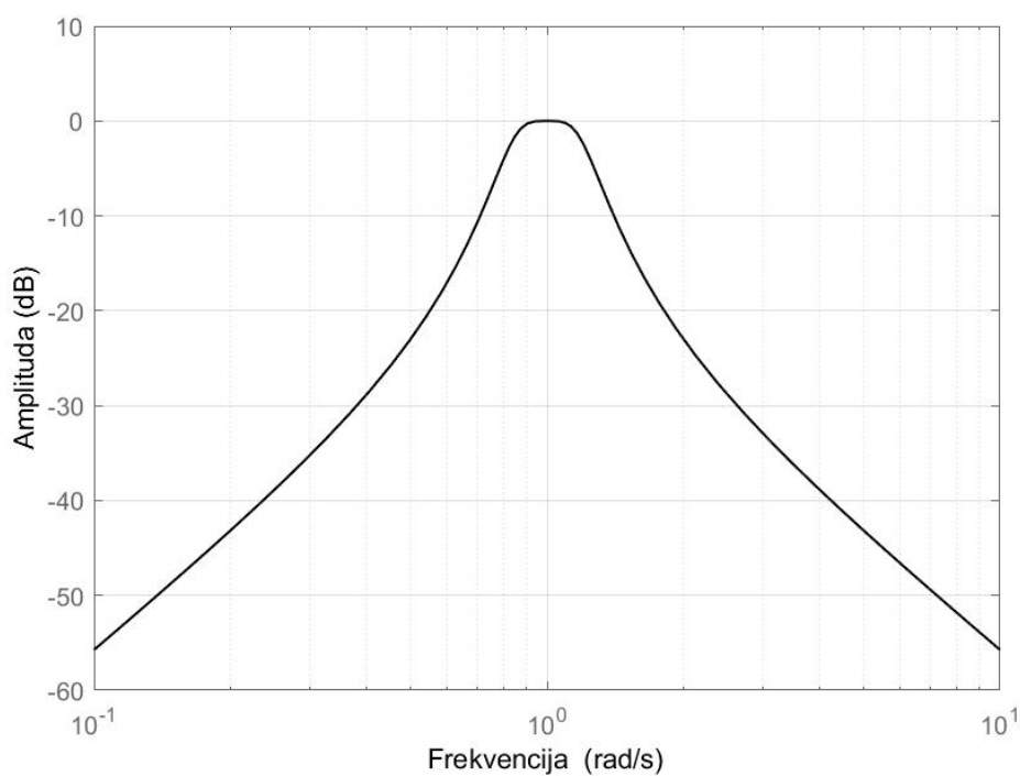
Slika 3.5. Normirana ukupna amplitudno frekvencijska karakteristika kaskade i kaskade bikvarta u logaritamskom mjerilu
