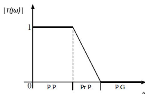
Slika 2.1 Amplitudno frekvencijska karakteristika NP filtra [1]
