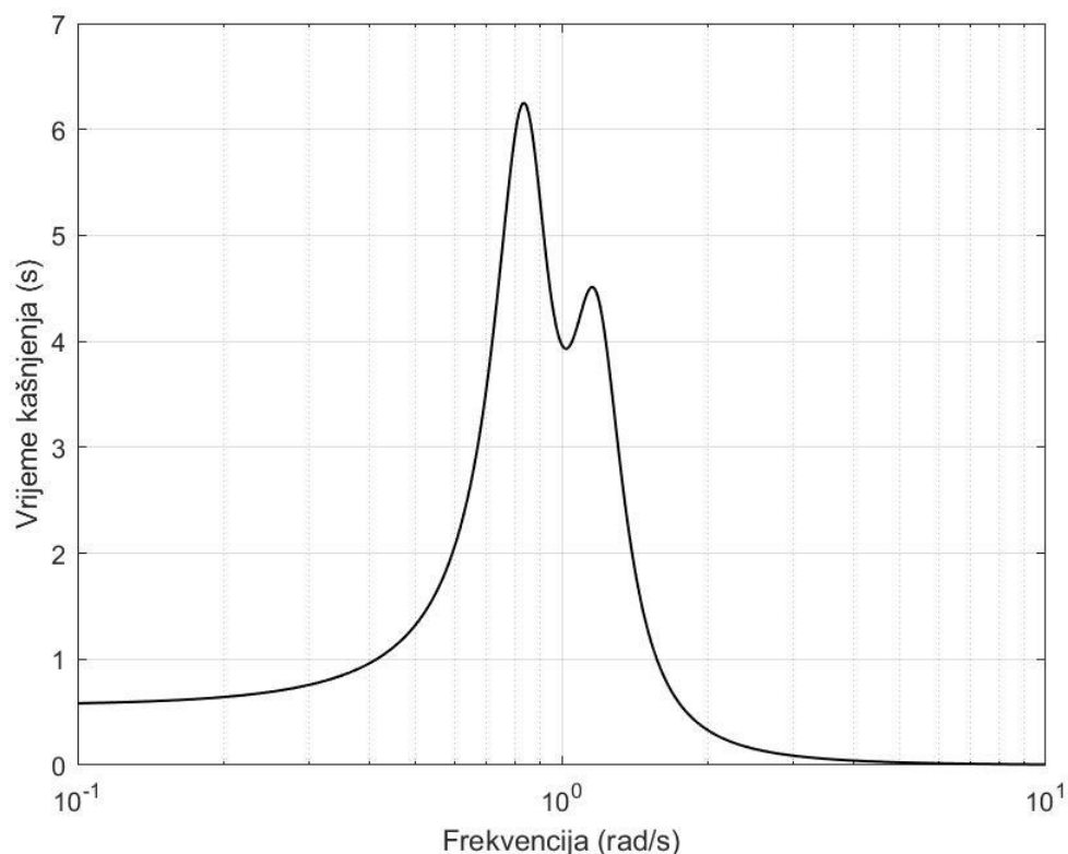
Slika 3.9. Normirana karakteristika grupnog vremena kašnjenja kaskade i kaskade bikvarta
