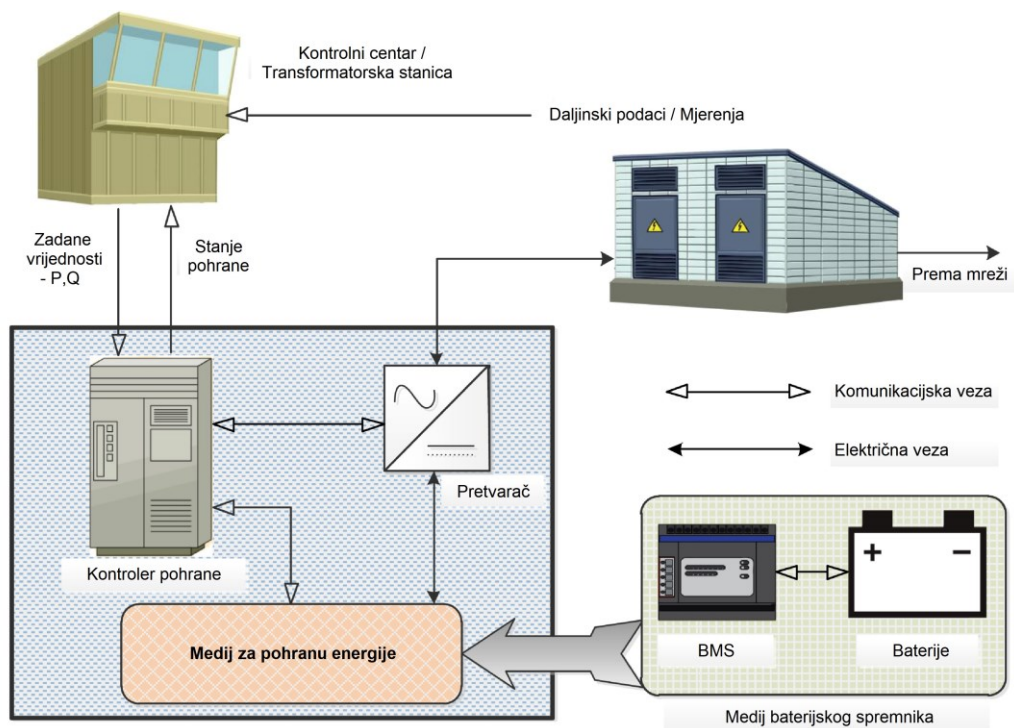
Slika 2.11. Baterijski spremnik energije (sustav) [17]
