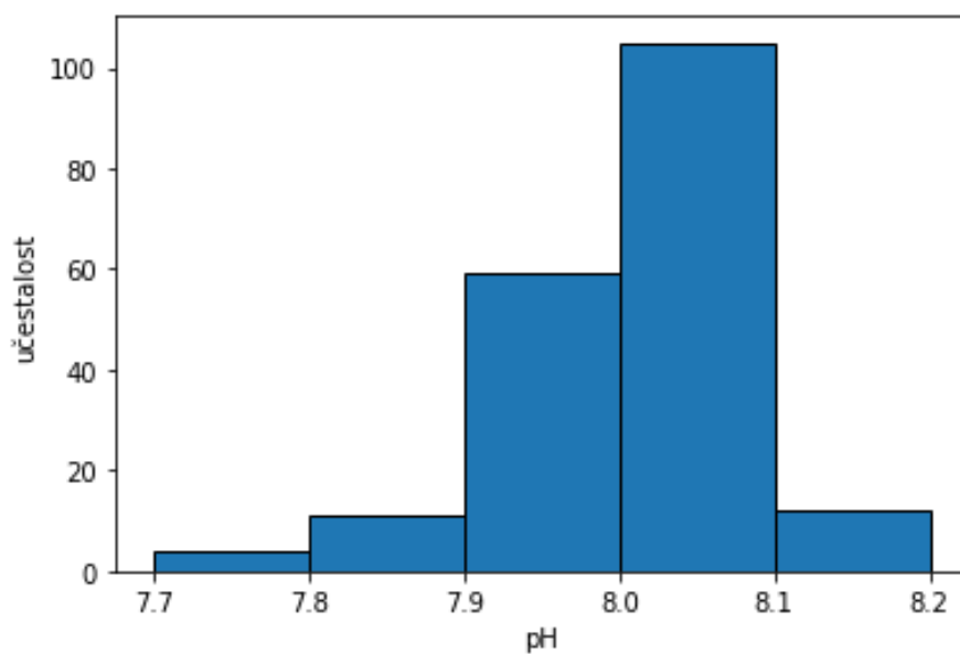
Slika 8.18: Raspodjela pH
