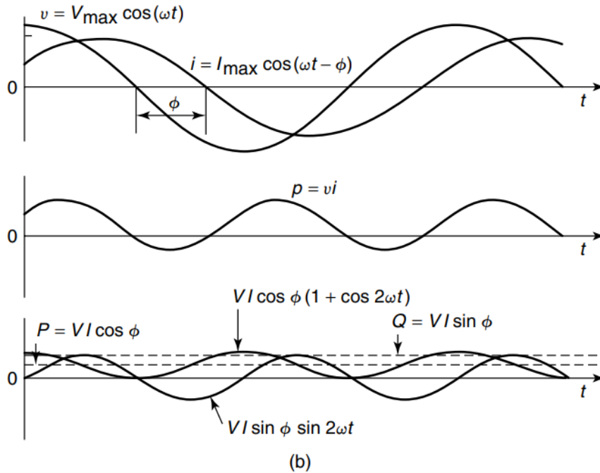
Slika 2.1. Parametri izmjeničnog strujnog kruga [2]
