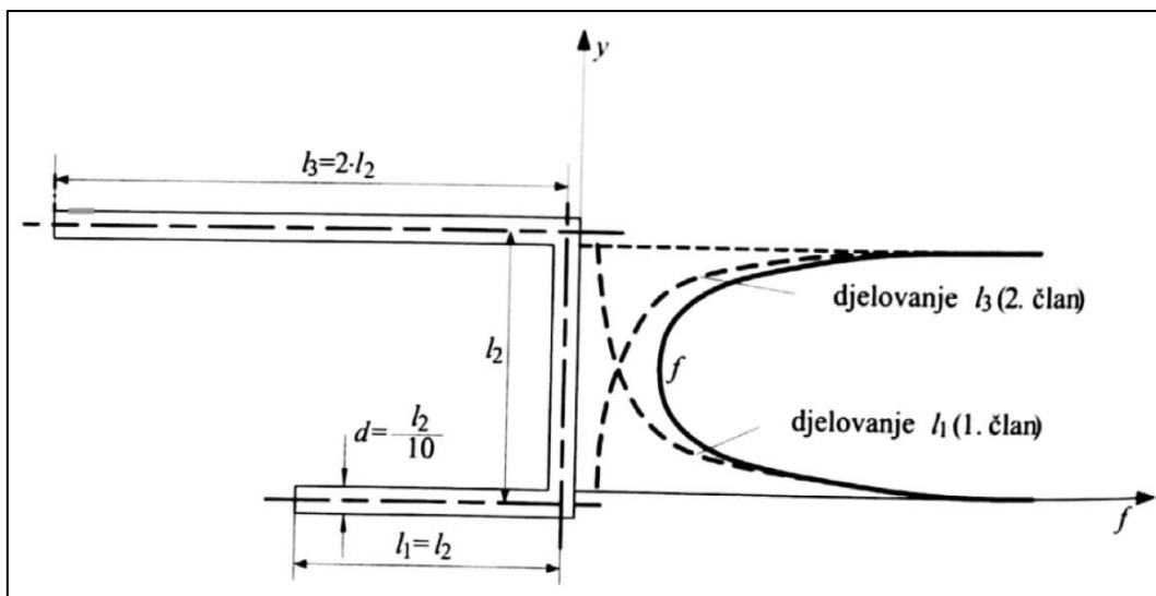
Slika 4.10. Sile po jedinici duljine f_{ds} i f_{\infty} na okomiti dio vodiča u obliku slova "U" [4]
