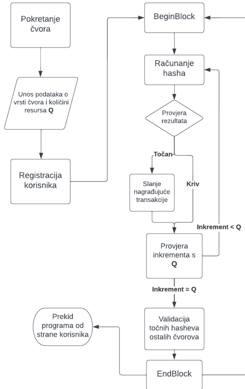
Slika 5.5 UML dijagram procesa u decentraliziranoj aplikaciji
