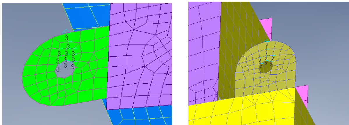
Slika 6.16. Postavljeni oslonci
