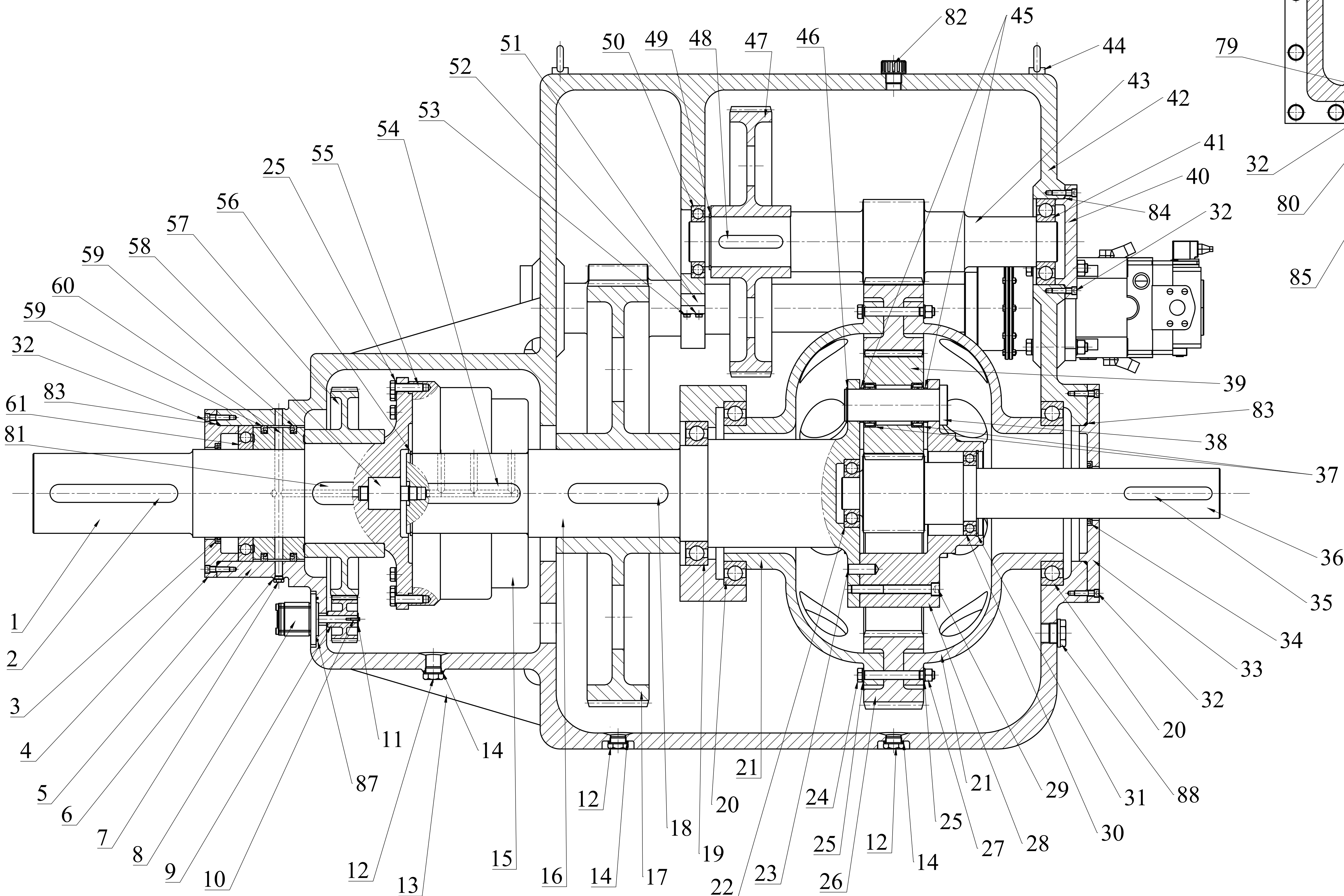
Presjek A-A
