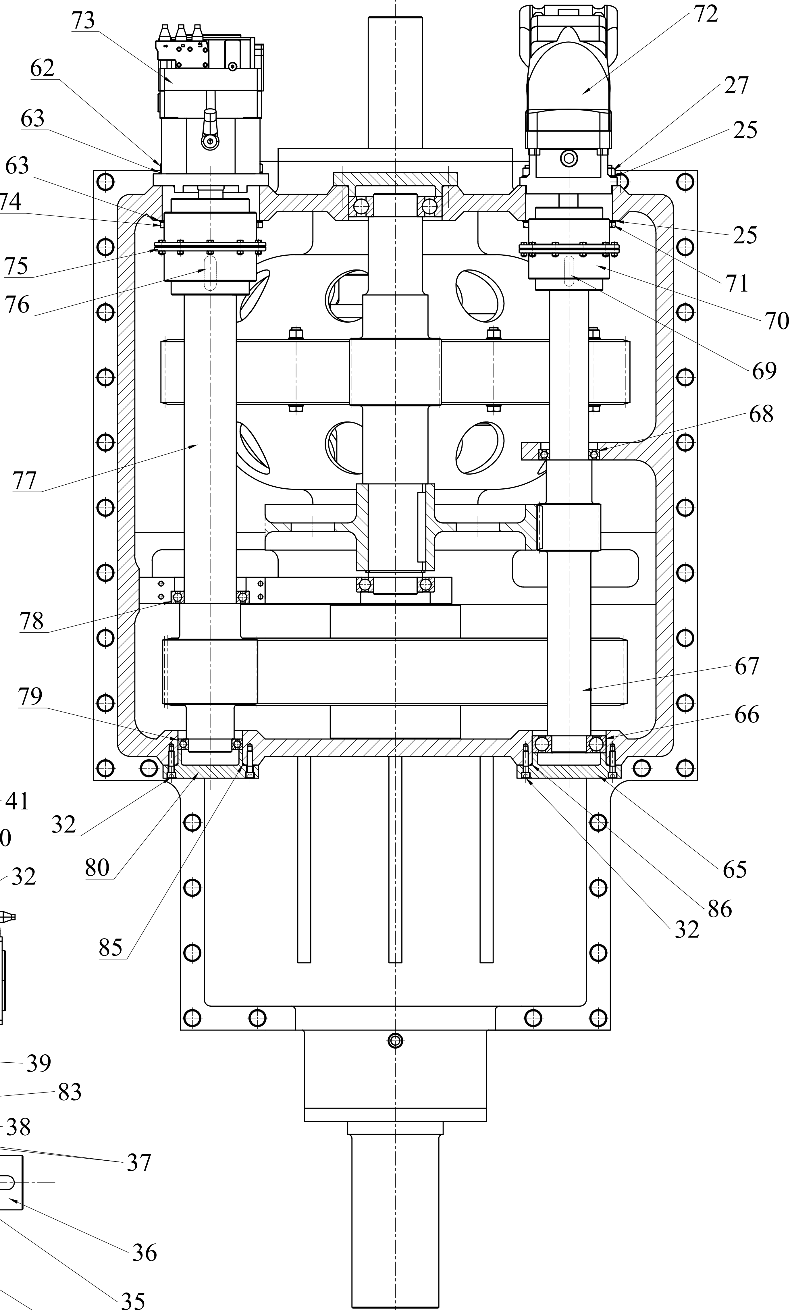
Presjek B-B
