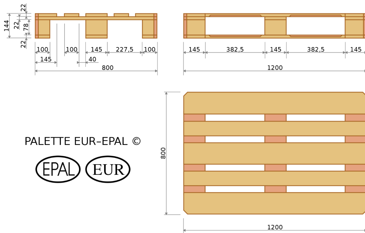
Slika 5.1 Dimenzije EUROPALETE [14]
