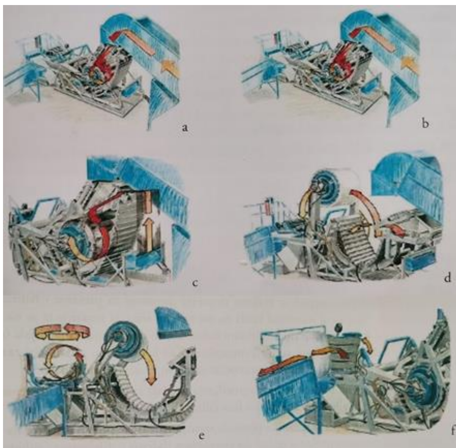
Slika 4.1 Prikaz postupka baliranja otpada [5]
