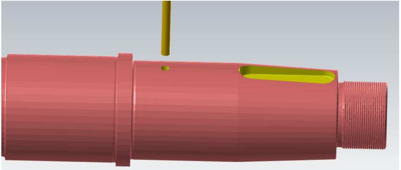
Slika 6.120 Simulacija operacije 50
