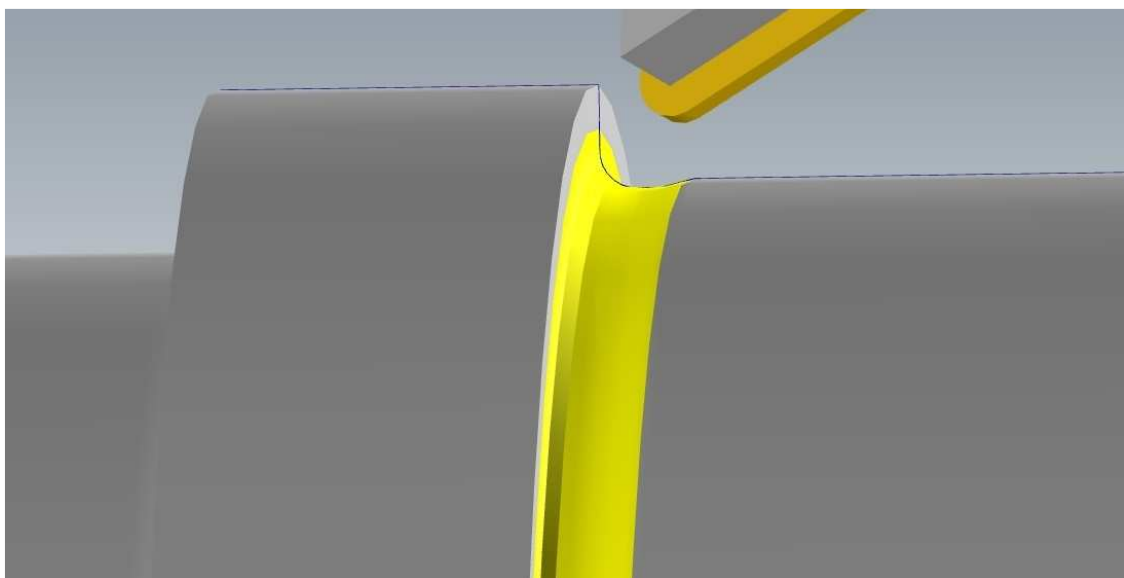
Slika 6.65 Zahvat 19 - Simulacija
