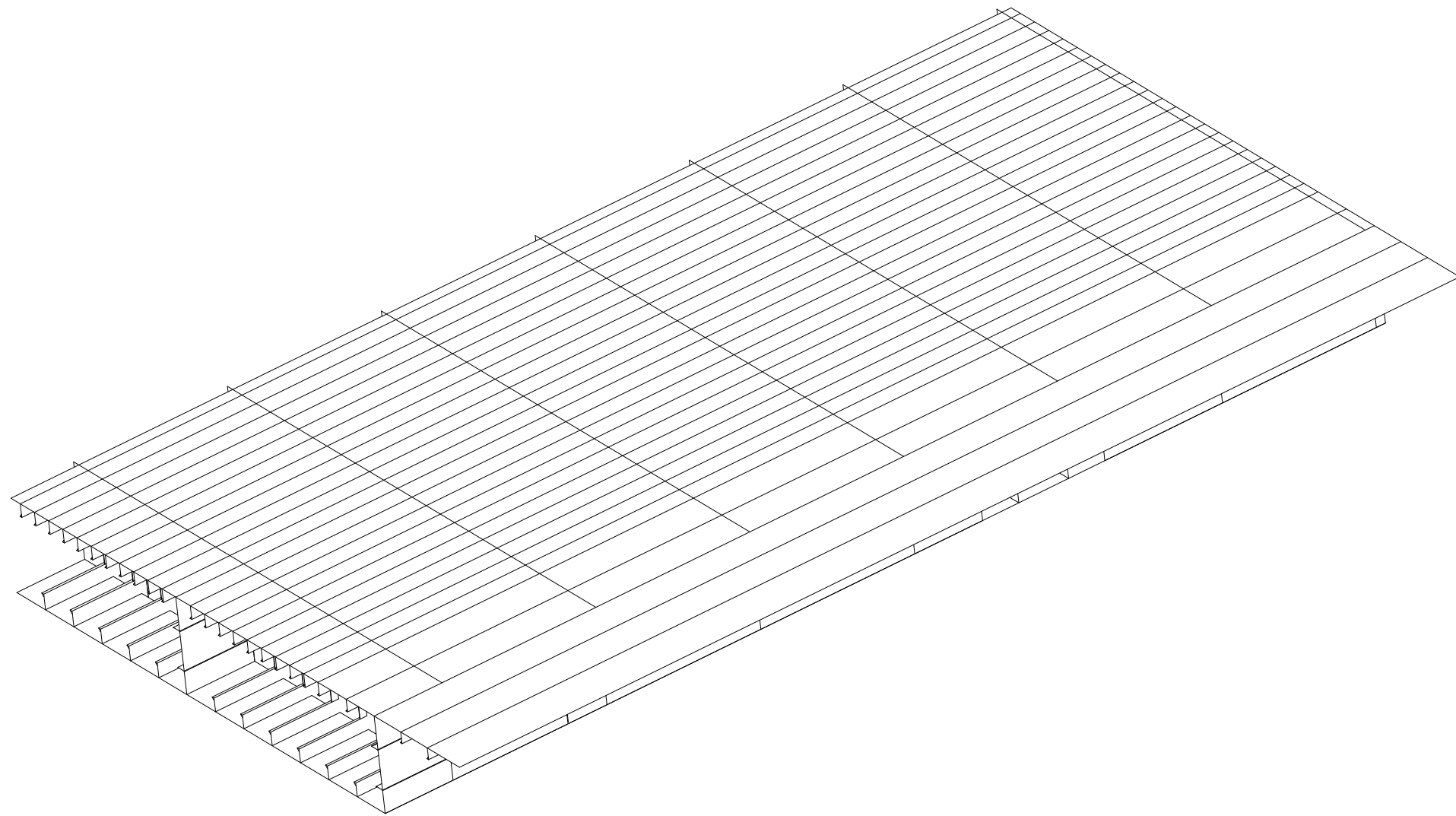
7. PANEL VANJSKE OPLATE SA UZDUŽNJACIMA + KOMPLETIRANI PANEL UZDUŽNE PREGRADE
