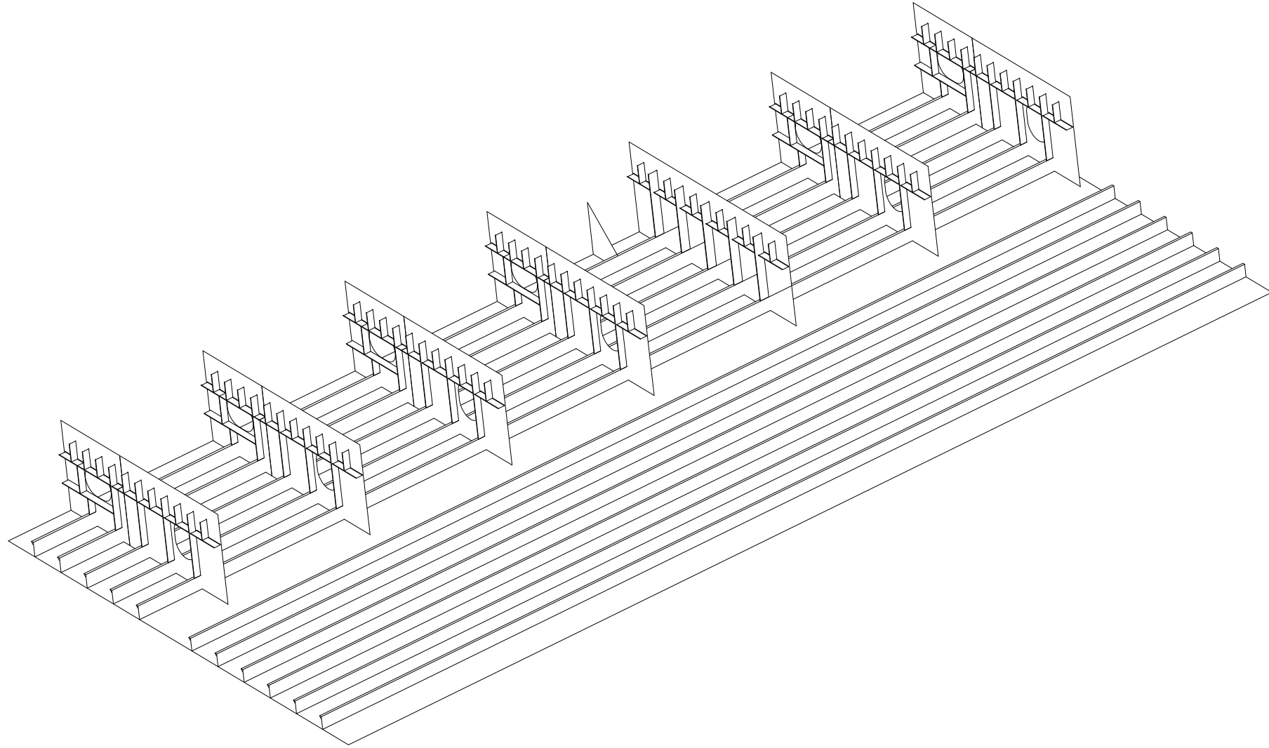
3. PANEL UZDUŽNE PRGRADE DVOBOKA + ELEMNTI REBRENICA + PROVEZA na 9860mm
