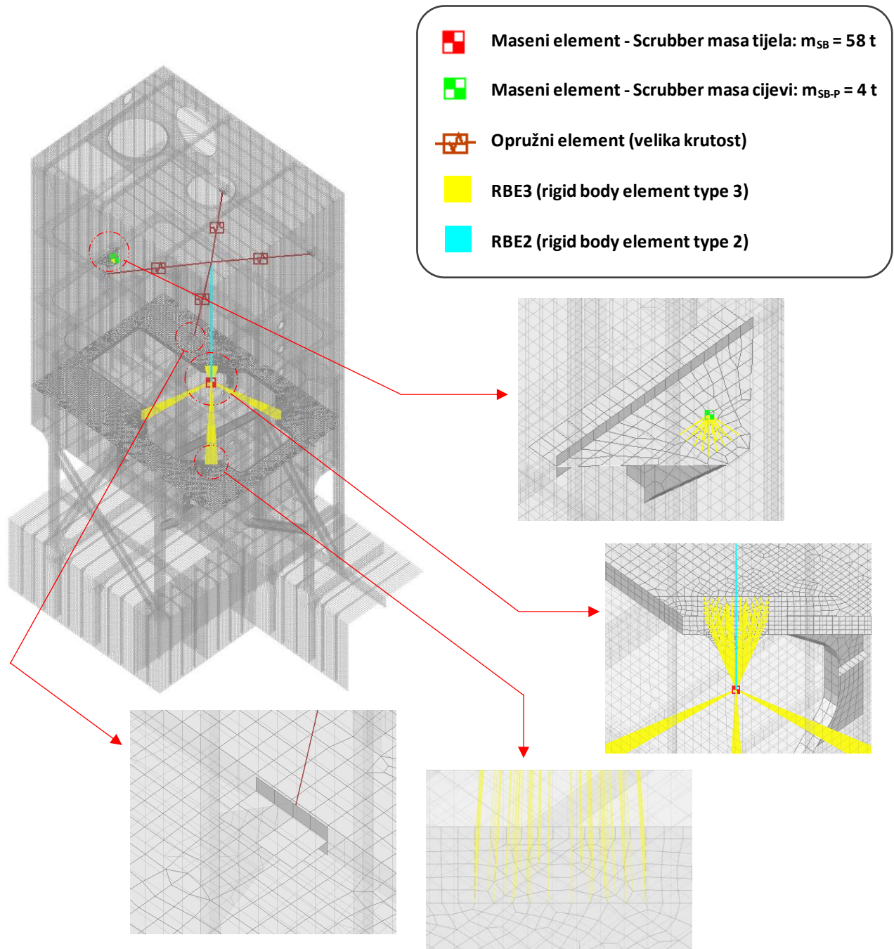
Slika 4.4. Primjer pripremljenog modela za FEA [4].
