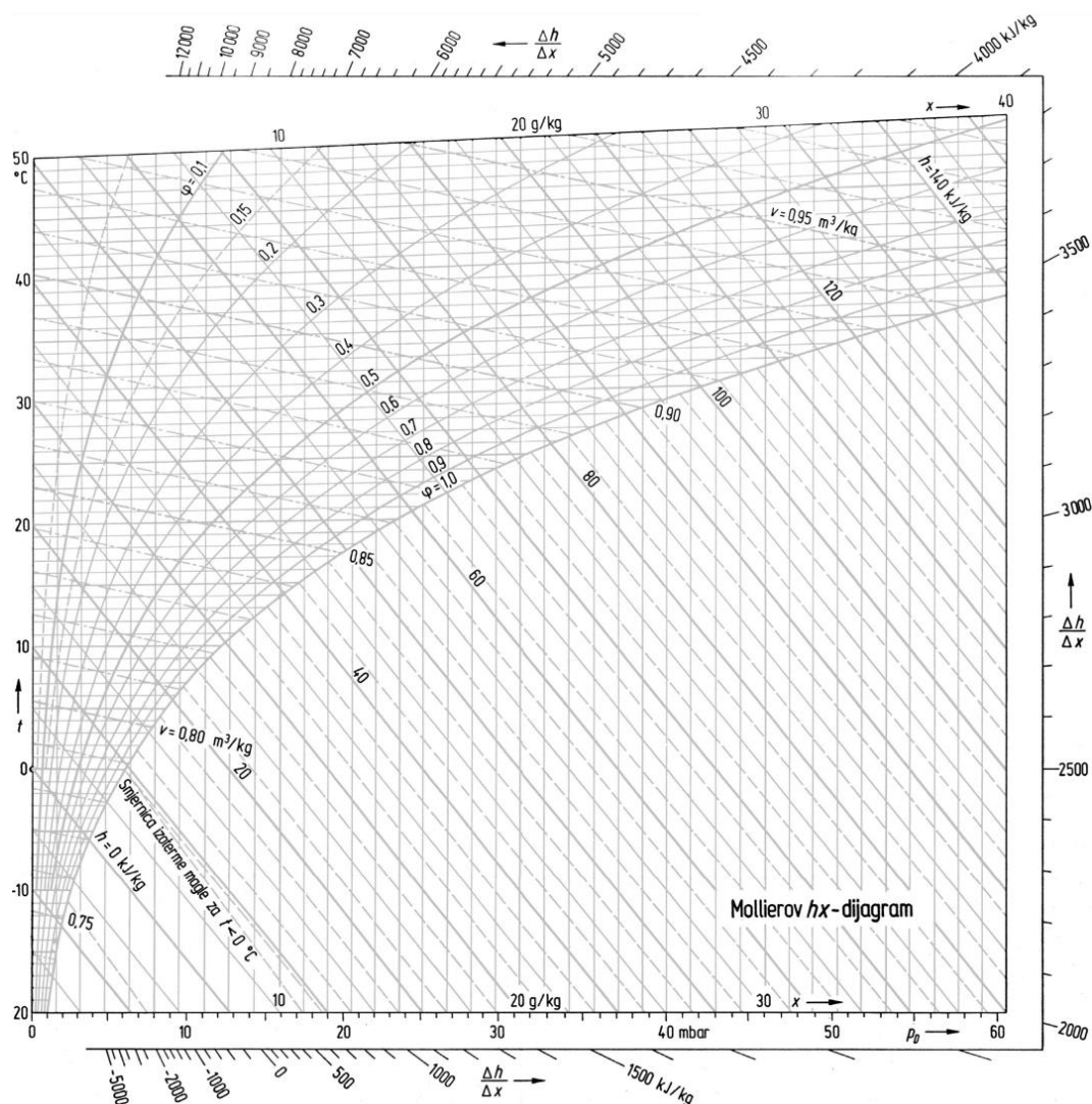
Slika 2.1 Mollierov hx – dijagram
