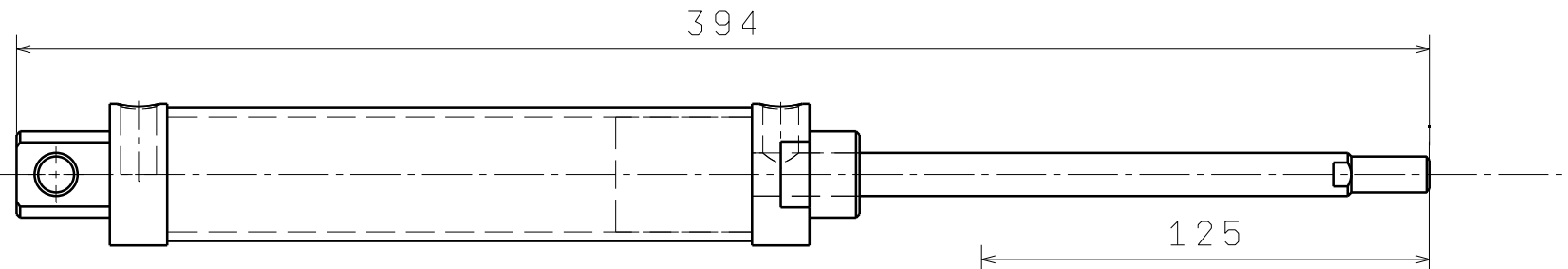
Prikaz ispruženog cilindra M 1:2
