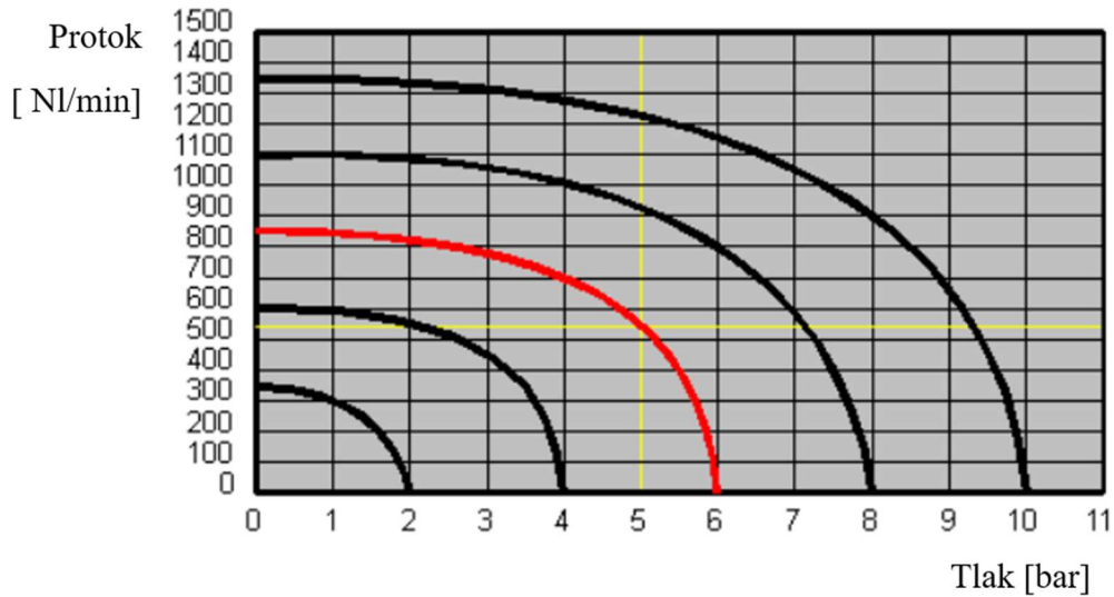
Slika 6.14. Zavisnost protoka o tlaku unutar razvodnog ventila [15]
