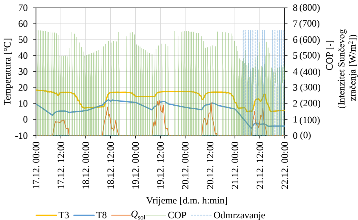
Slika 8.2 Vremenske promjene temperature akumulatora topline (T3), temperature okolišnjeg zraka (T8), trenutnog COP-a dizalice topline i trenutnog intenziteta sunčevog zračenja (Q sol ) od 17.12. do 22.12. za optimalnu konfiguraciju sustava A ( V = 2,5 \text{ m}^3 , A = 46,4 \text{ m}^2 , T_l = 19 \text{ °C} )
