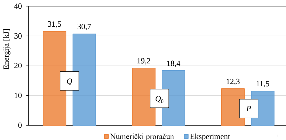
Slika 5.18 Usporedba izmijenjenih toplina u kondenzatoru (Q), isparivaču (Q 0 ) i utrošenih električnih energija za pogon dizalice topline (P) dobivenih numeričkim i eksperimentalnim putem za protok vode kroz kondenzator 4700 kg/h, protok vode kroz isparivač 9620 kg/h i početnu temperaturu vode 23 °C
