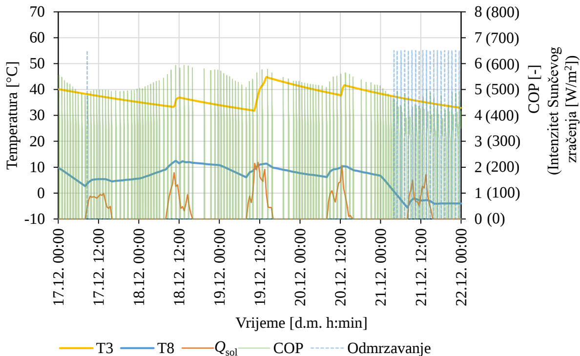
Slika 8.3 Vremenske promjene temperature akumulatora topline (T3), temperature okolišnjeg zraka (T8), trenutnog COP-a dizalice topline i trenutnog intenziteta sunčevog zračenja (Q sol ) od 17.12. do 22.12. za optimalnu konfiguraciju sustava B ( V = 2,5 \text{ m}^3 , A = 46,4 \text{ m}^2 , T_l = 54 \text{ °C} )
