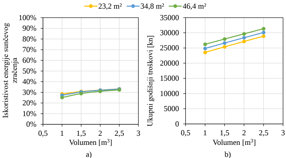
Slika 7.18 Ovisnost iskoristivosti energije sunčevog zračenja (a) i ukupnih godišnjih troškova (b) o volumenu latentnog spremnika topline za Sustav B, za različite površine solarnih kolektora 23,2 m², 34,8 m² i 46,4 m² i za temperaturu taljenja akumulatora topline 54 °C
