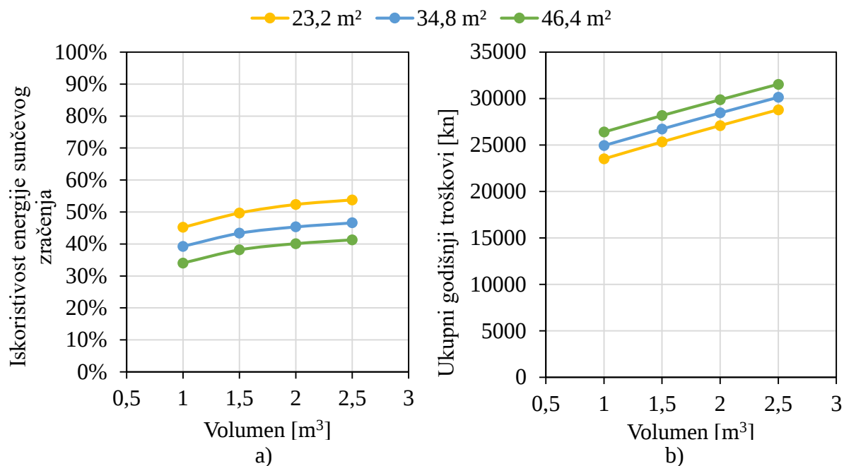
Slika 7.9 Ovisnost iskoristivosti energije sunčevog zračenja (a) i ukupnih godišnjih troškova (b) o volumenu latentnog spremnika topline za Sustav A, za različite površine solarnih kolektora 23,2 m², 34,8 m² i 46,4 m² i za temperaturu taljenja akumulatora topline 19 °C
