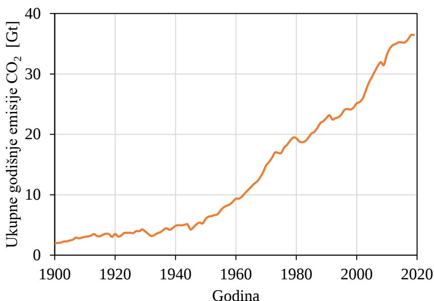
Slika 1.1 Porast ukupne godišnje emisije \text{CO}_2 tijekom 20. i početkom 21. stoljeća [1]
