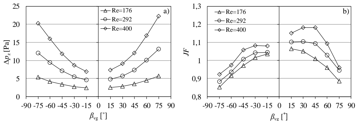
Slika 7.12. Usporedbe koeficijenta prijelaza topline na strani zraka a) i udjela toplinskih otpora na strani zraka u ukupnom otporu prolazu topline b) za analizirane upadne kutove generatora vrtloga
