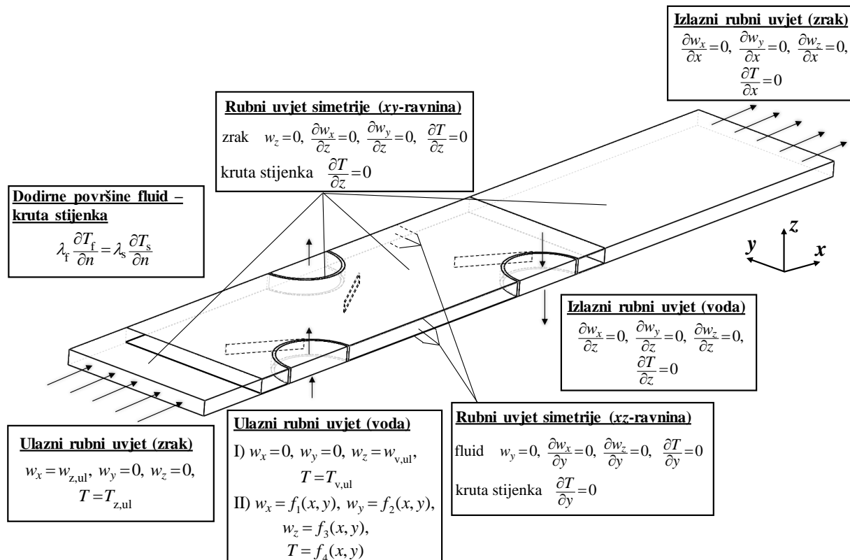
Slika 3.3. Proračunska domena s pripadajućim rubnim uvjetima
