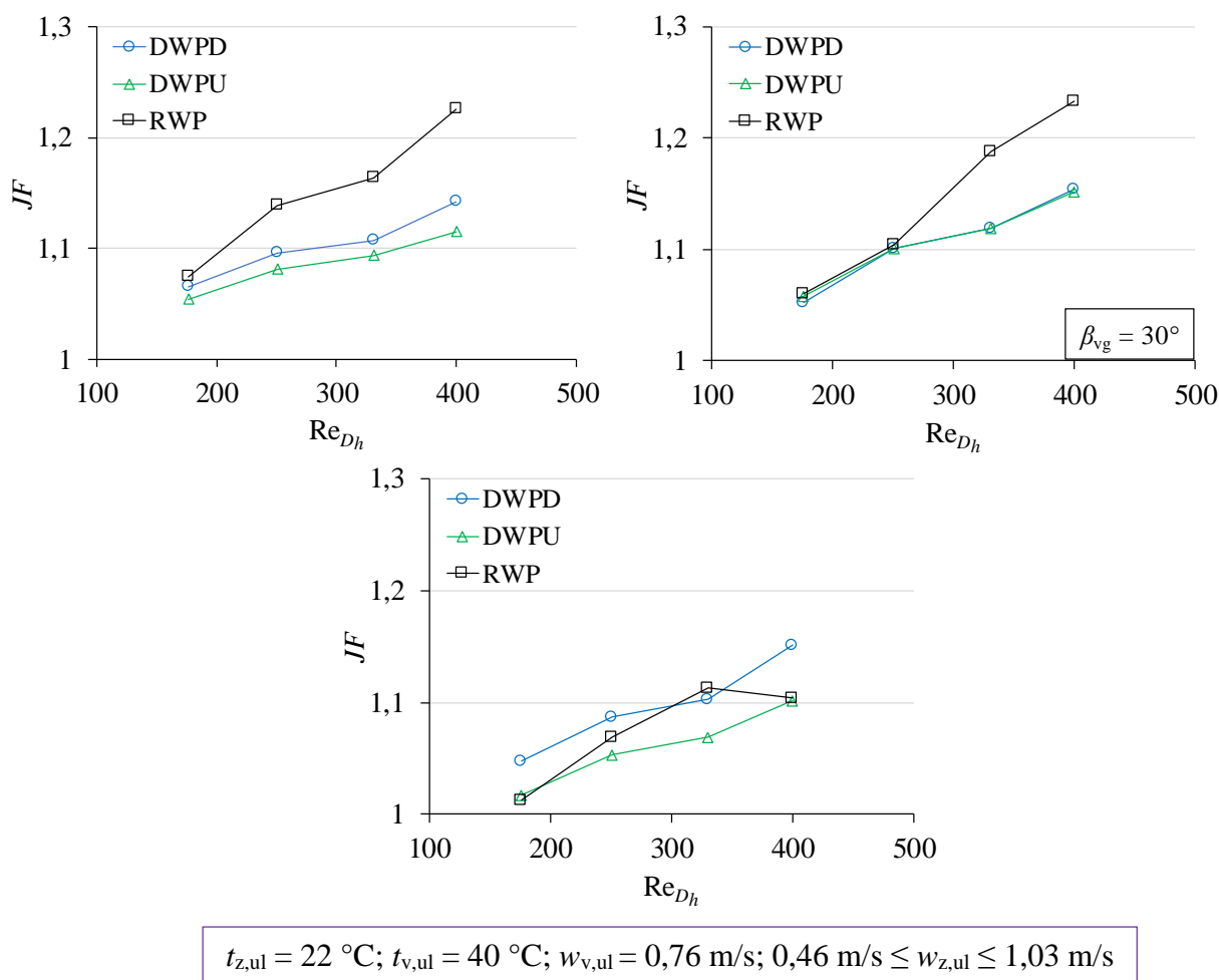
Slika 7.9. Usporedba JF faktora za cijevne lamelne izmjenjivače topline s pravokutnim krilcima (RWP), nizvodnim delta krilcima (DWP) i uzvodnim delta krilcima (DWPU) pri različitim upadnim kutovima
