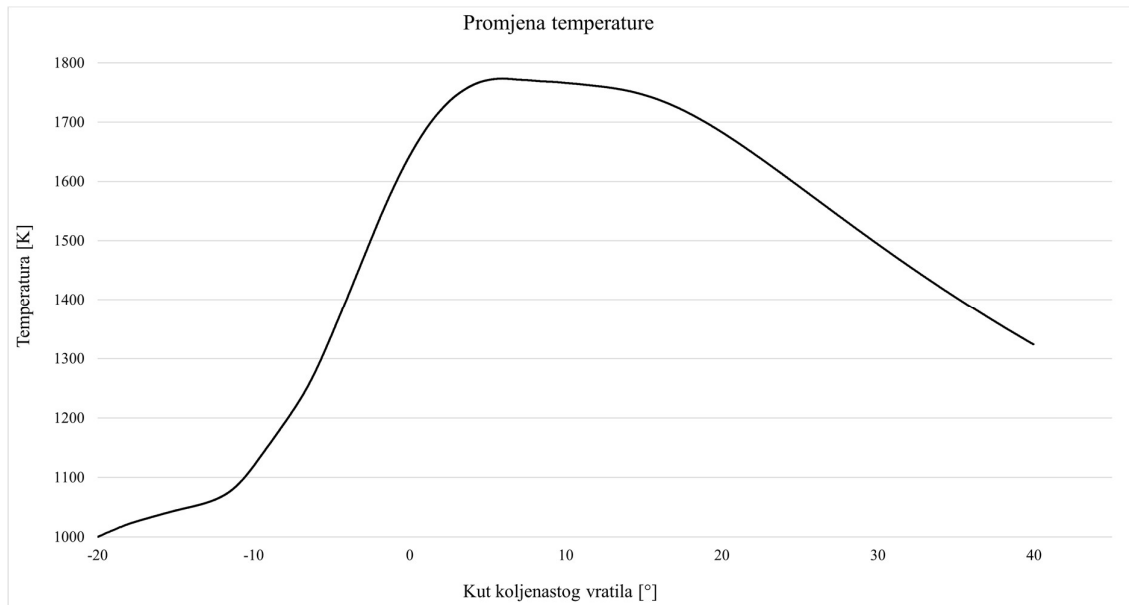
Slika 8.1. Promjena temperature
