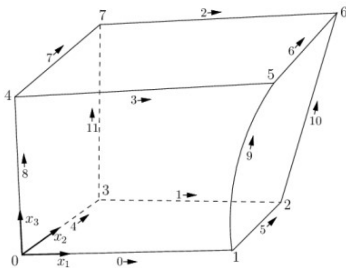
Slika 7.1. 3D heksaedarski blok [13]
