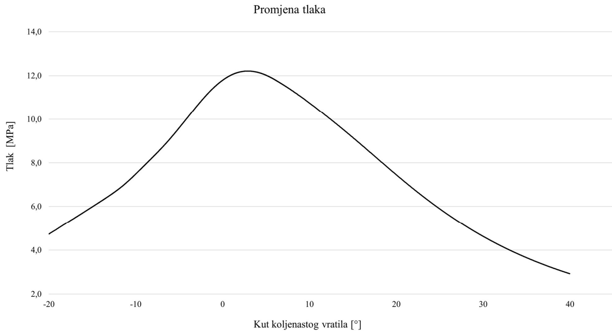
Slika 8.7. Promjena tlaka
