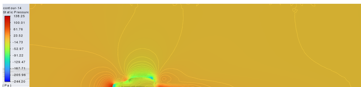
Slika 0.8 Kontura statičkog tlaka za ulaznu brzinu v = 15 \text{ m/s}
