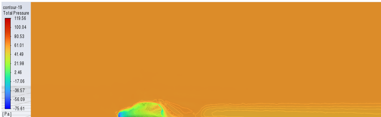
Slika 0.5 Kontura totalnog tlaka za ulaznu brzinu v = 10 m/s
