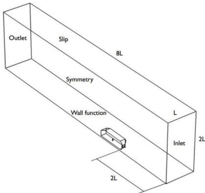
Slika 0.3 Smjernica za izradu domene
