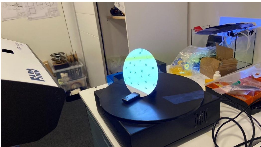
Slika 3.7 Kalibracija skenera
