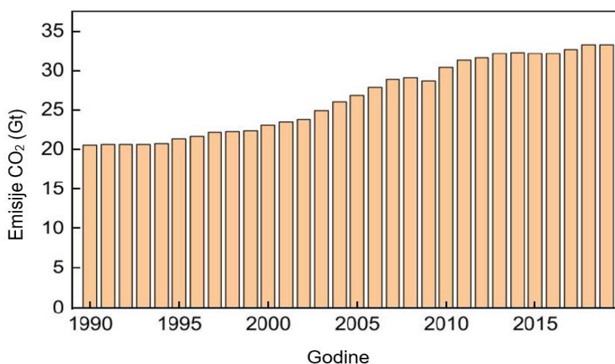
Slika 2.1. Emisije CO 2 povezane s energetske sektorom od 1990. do 2019. Godine [2]
