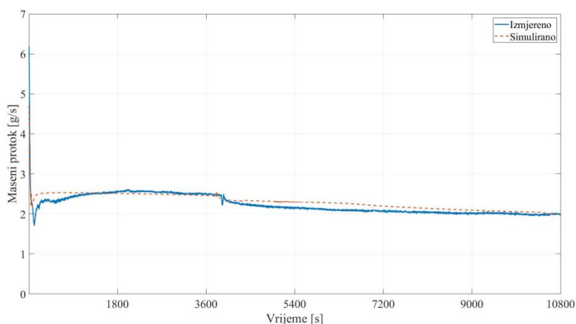
Slika 64. Maseni protok kroz kompresor (konfiguracija 170-24)
