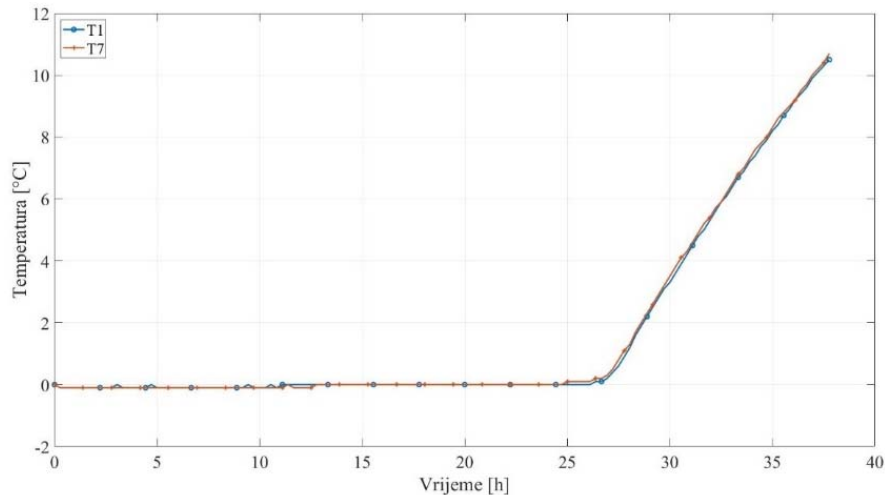
Slika 33. Temperatura rashladne kupke s uključenim mješačem
