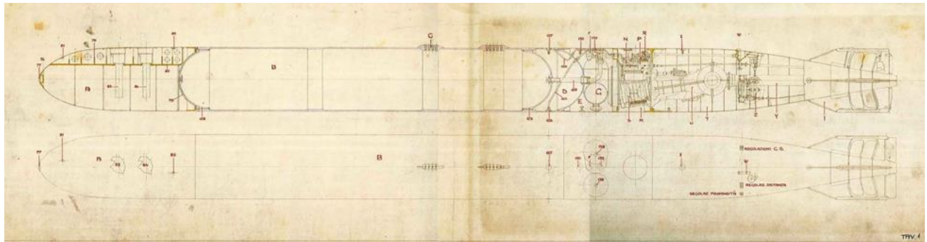
Slika 4.24. Skica – TR 53/IV torpedo
