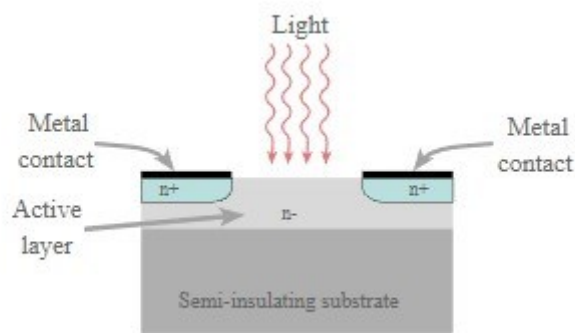
Slika 4.2: Struktura fotooptornika [9]
