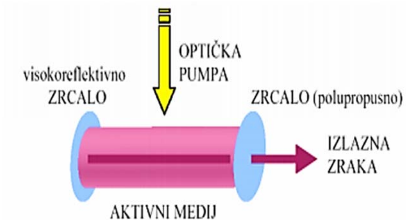
Slika 3.1. Dijelovi lasera [1]
