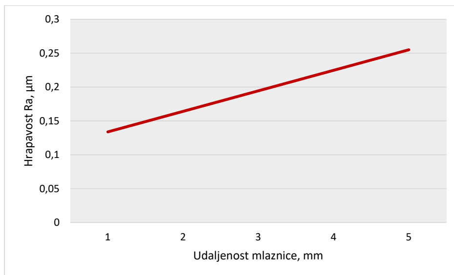
Slika 7.10. Grafički prikaz modela površinske hrapavosti
