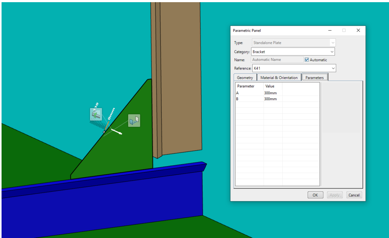
Slika 5.29. Koljeno „K41“
