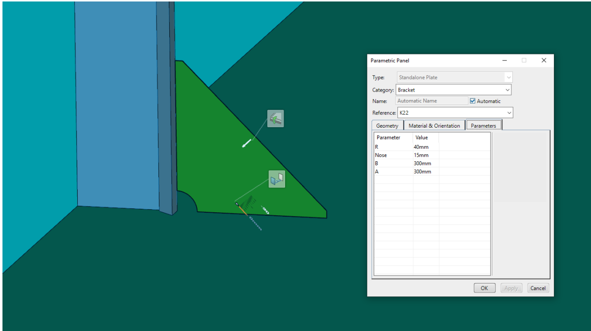
Slika 5.20. Koljeno „K22“
