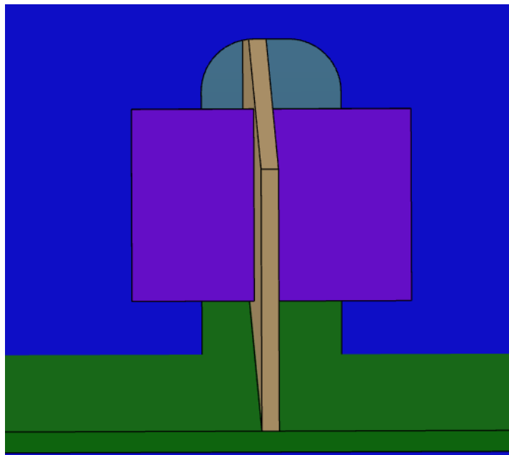
Slika 6.48. Prikaz prolaza profila „P12-FB150x10“ unutar detaljnog model broda
