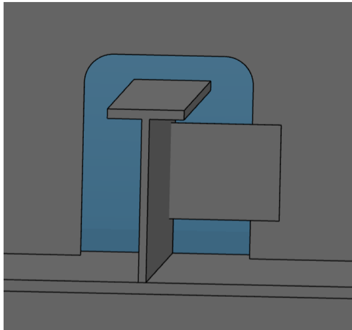
Slika 6.71. Prikaz prolaza profila „P21-TB180x8x80x10“ unutar detaljnog model broda
