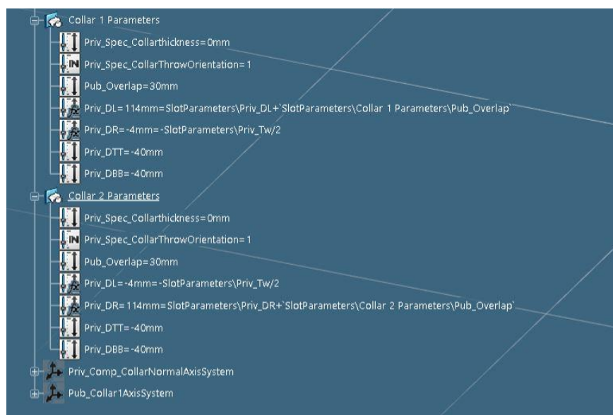
Slika 6.74. Parametri definicije konture generičkog prolaza profila „P21-TB180x8x80x10“, 3.dio
