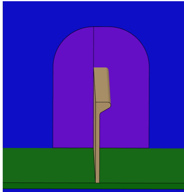
Slika 6.26. Prikaz prolaza profila „P5-HP160x8“ unutar detaljnog model broda
