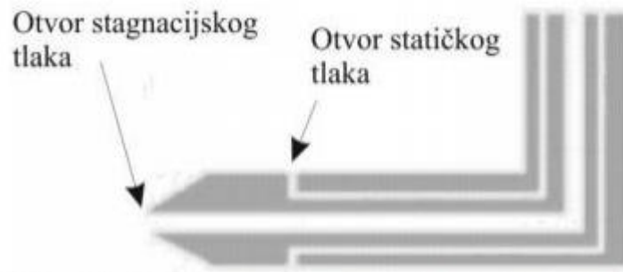
Slika 4.4. Pitotova cijev mjeri stagnacijski i statički tlak [4]
