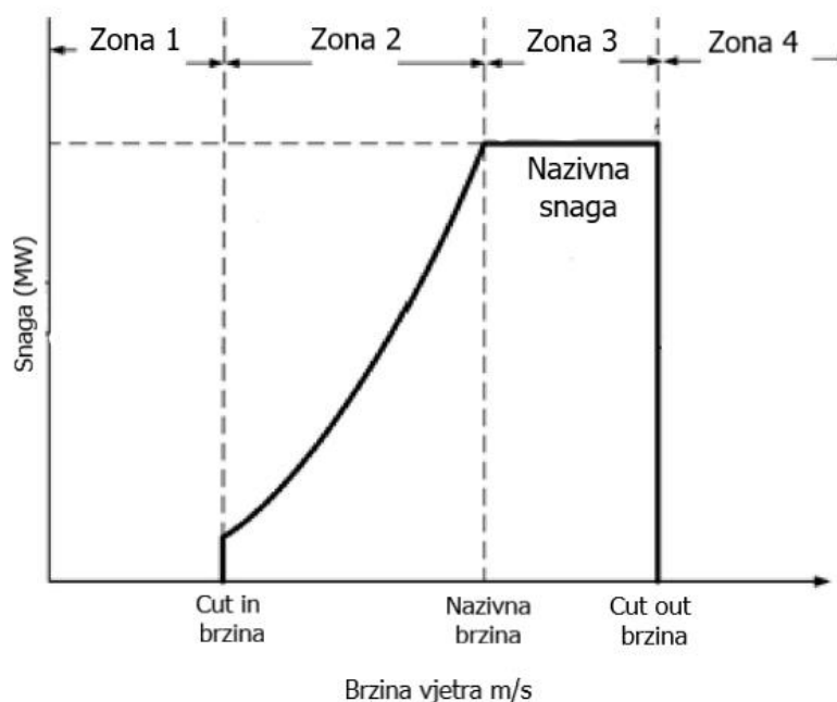
Slika 3.9. Radna područja vjetroatogregata
