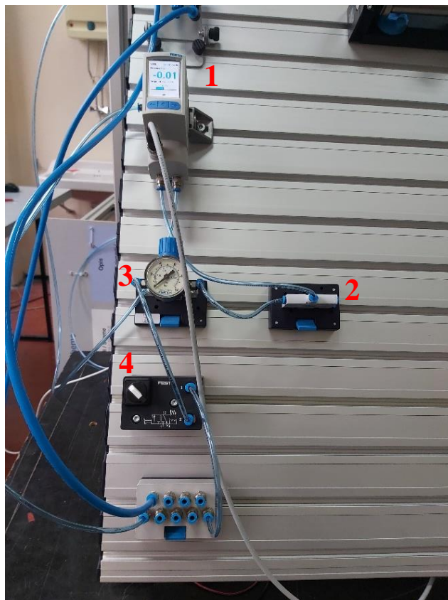
Slika 5.1 Pnevumatska oprema
