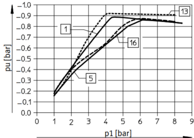
Slika 5.3 Ovisnost generiranog podtlaka o ulaznom pretlaku [22]
