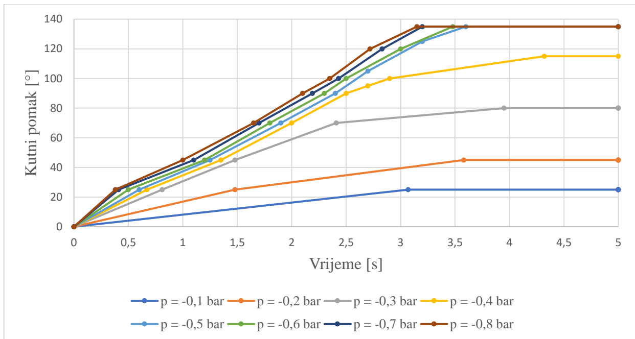
Slika 6.14 Mjerenje vremena ostvarivanja određenog kutnog pomaka pri različitim vrijednostima podtlaka s opterećenjem od 0,55 kg
