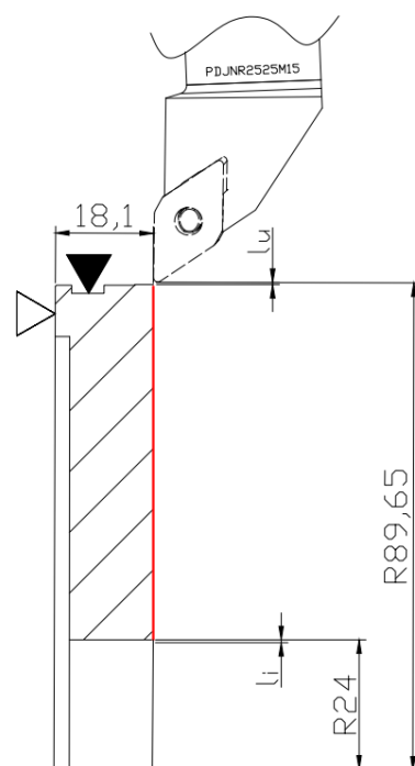
Slika 5.36. Operacija 40 – zahvat 2
