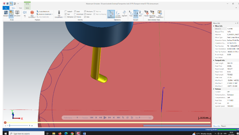
Slika 7.131. Simulacija (OP150)
