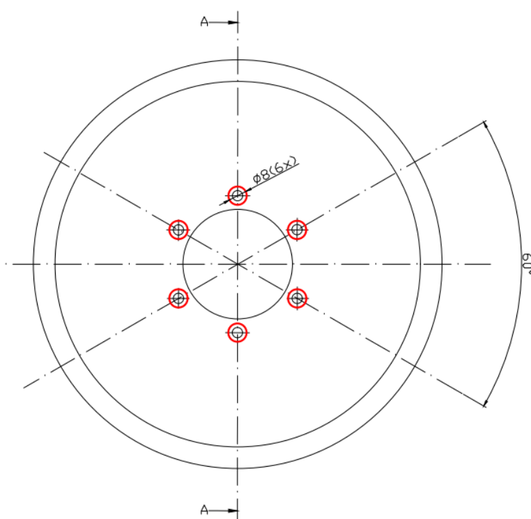
Slika 5.56. Operacija 50 - zahvat 5
