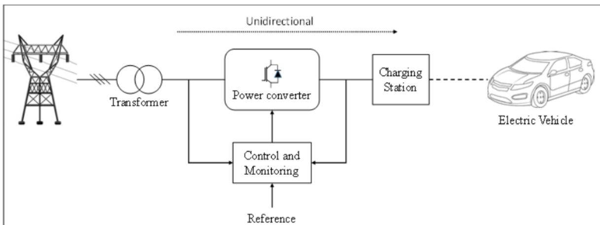
Slika 5.1.1. Prikaz funkcionalnosti G2V sustava [15]
