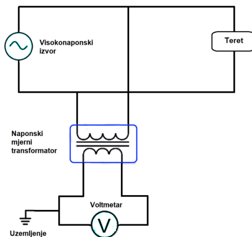
Slika 3.6. Paralelni spoj naponskog mjernog transformatora
